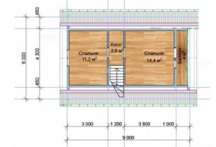
Проект №07: Дом из бруса 6х6 м с мансардой и террасой 6х3 м
