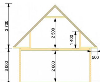
Проект №07: Дом из бруса 6х6 м с мансардой и террасой 6х3 м
